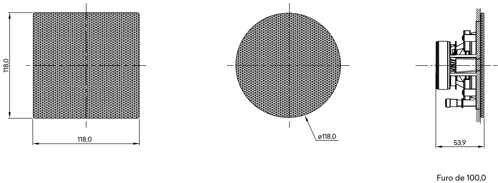
Dimensões - 75121 | 75122 (mm)
