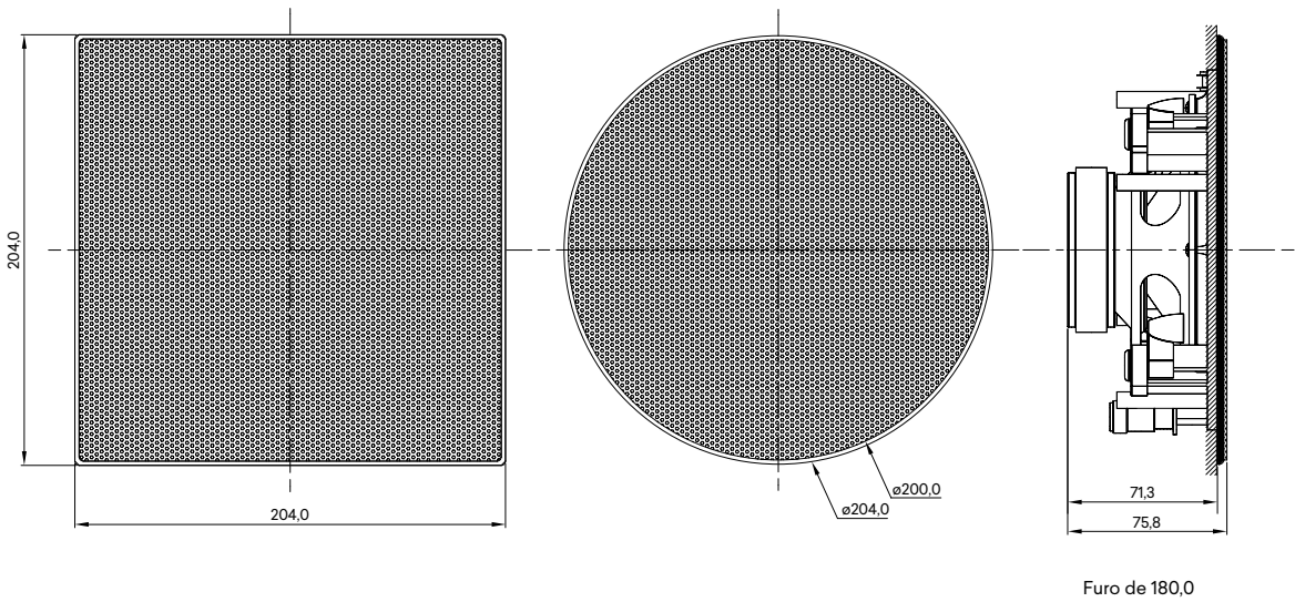
Dimensões - 75104 C | 75105 C (mm)
